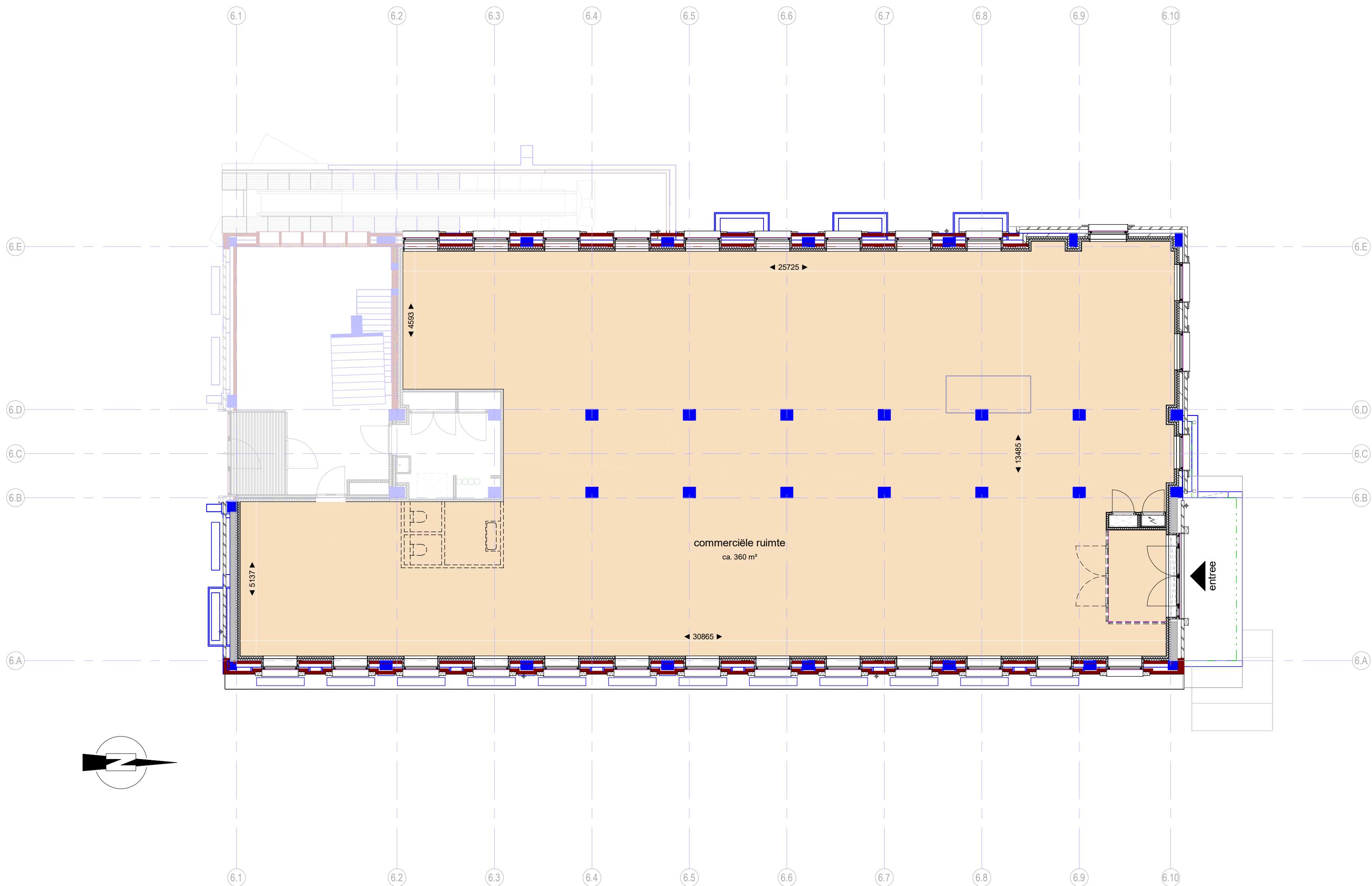
begane grond 1 : 100
